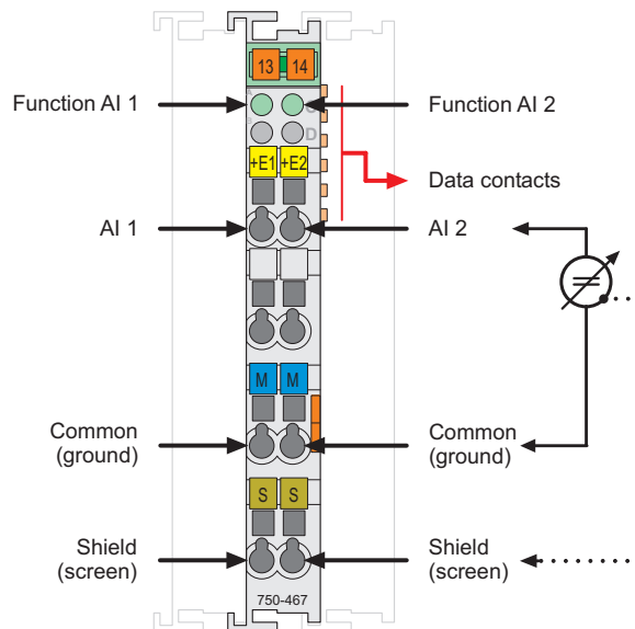
Fig. 2.1.1-1: 2-Channel Analog Input Module 750-467
